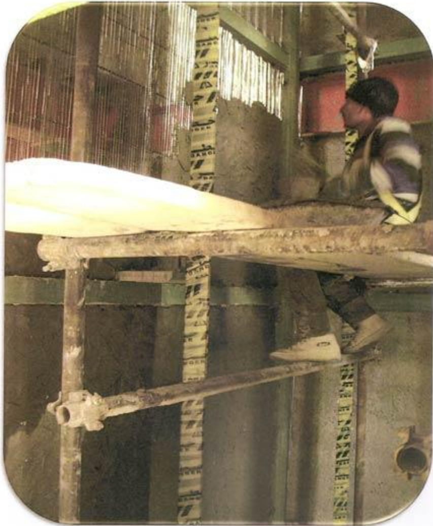
اجرای آستر سیمان روی دیوار چایی آستانور
